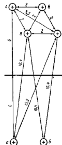
Рис. 14. Схема расположения проводов
